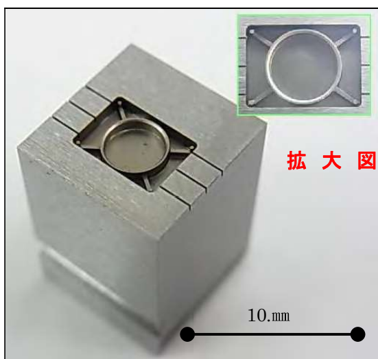
材質 SKH51 (62HRC) 使用機械 EA8PV (三菱) 放電面 面粗度 Rz\ 1.00\ \mu m 細溝 3本放電仕上げ 幅 0.10 深さ 0.5
