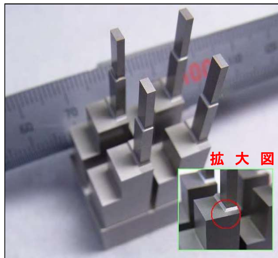
材質 DC 53 (58HRC) 使用機械 FA10P (FS電源加工) 面粗度 Ra\ 0.22\ \mu m 2方向から加工 合わせ段差 \pm 0.005
