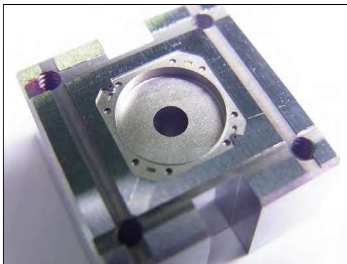
材質 PD613 (58~60HRC) 使用機械 EA8PV (三菱) 放電面 面粗度 Rz\ 1.00\ \mu m
